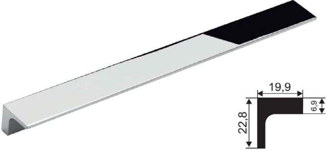
Alüminyum MS-0475 Geniş L Krom / İnox 96 / 128 / 160 / 192 / 224 / 320 mm
